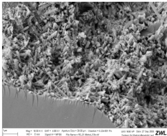
Nella foto ottenuta al microscopio si evidenzia il fittissimo legame tra il supporto e i prodotti di idratazione del cemento sinonimo di elevata adesione.
